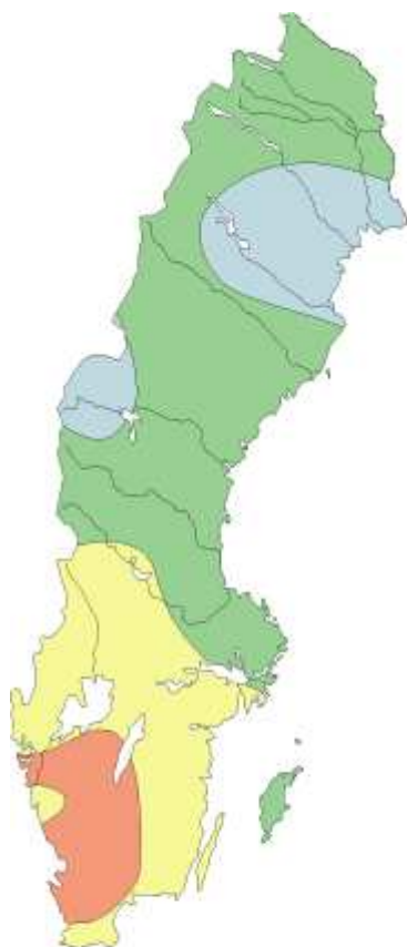
Grundvattennivåer
